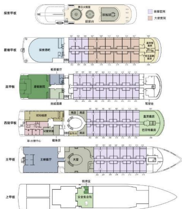
長江探索號樓層甲板圖
